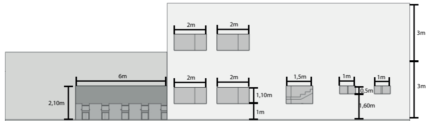
FACHADA NORTE
