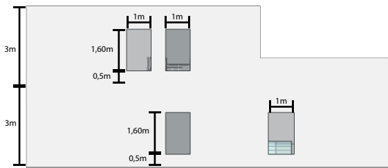
FACHADA OESTE
