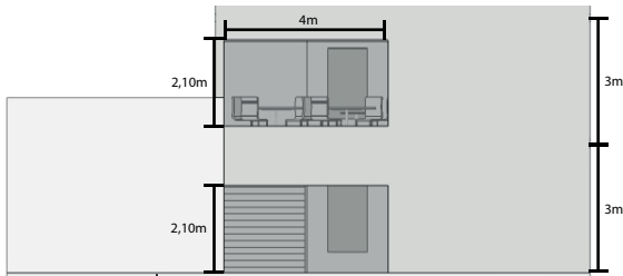
FACHADA LESTE
